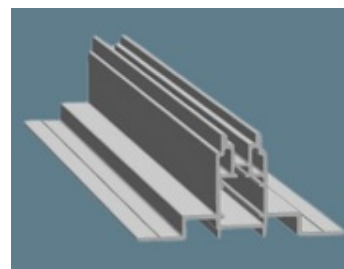
SISO 4K Standbauschienen 80x80 Alu Blank 5.40m SKU: 200.024 CHF 228.80
